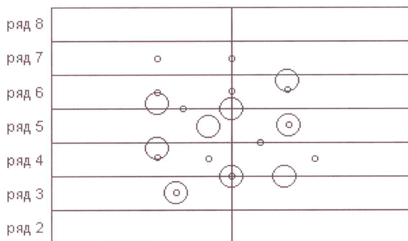
Рис. 1. Вид фрагмента стены с теплой стороны, охваченного датчиками теплового потока.
